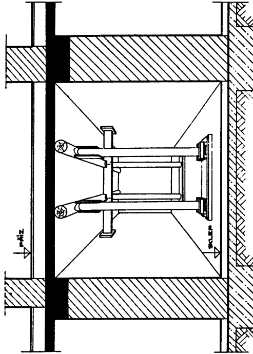
PERSPEKTIVNÍ POHLED
